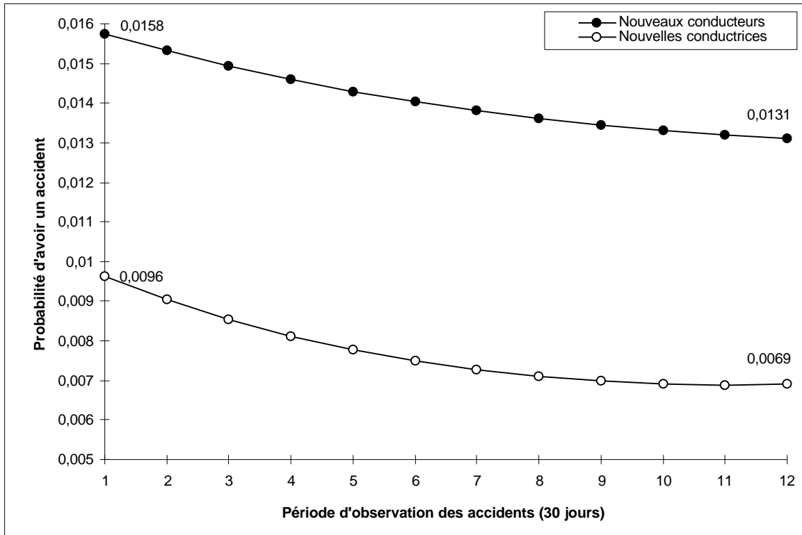
Figure 1: Probabilités d'avoir un accident au cours de 30 jours, estimées à l'aide du modèle 6, pour une période d'un an suivant la date d'obtention du permis.
