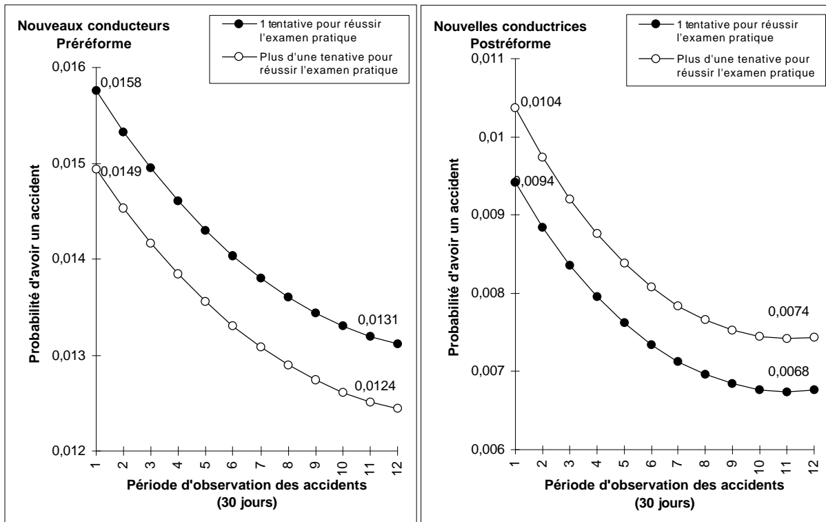
Figure 2: Probabilités d'avoir un accident au cours de trente jours, estimées à l'aide du modèle 6, selon le nombre de tentatives pour réussir l'examen pratique, pour les nouveaux conducteurs de la préréforme (à gauche) et pour les nouvelles conductrices de la postréforme (à droite).
